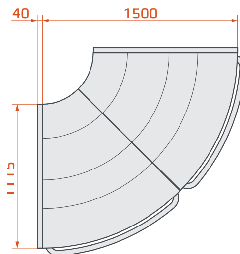
INT 2x45°
